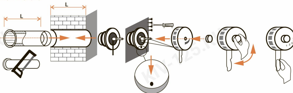
Рис. 3 - Монтаж клапана
