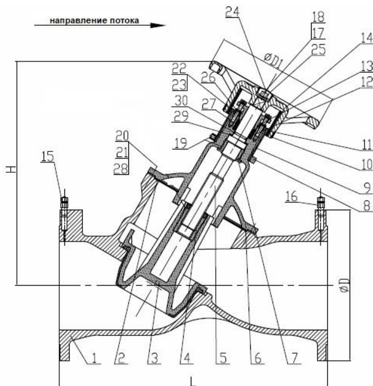
Рис.2. Клапан балансировочный фланцевый Ду200-Ду600.
