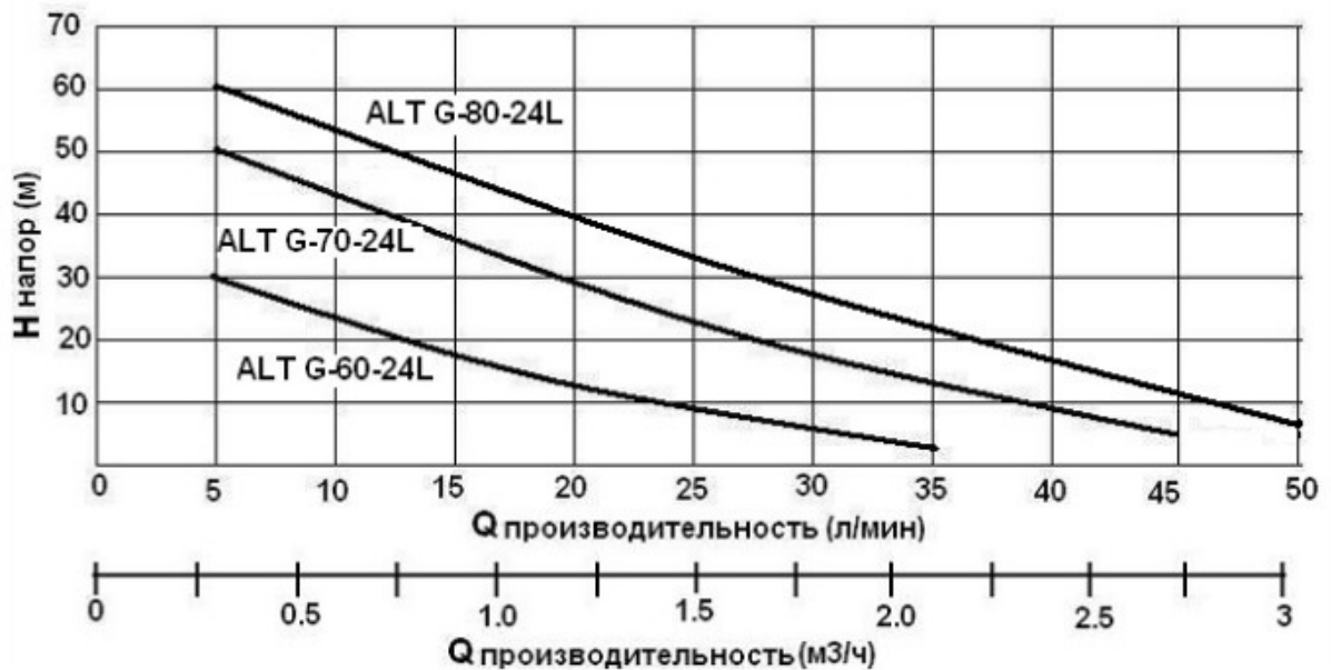
Диаграмма напорно-расходных характеристик
